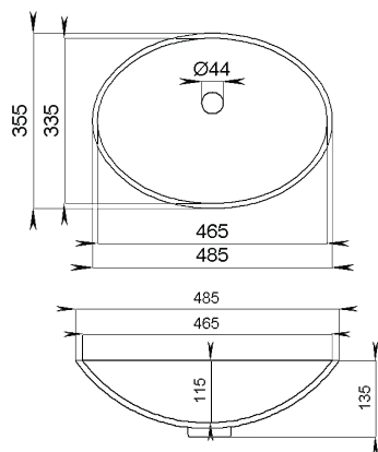
Модель ГС ОВП -465
