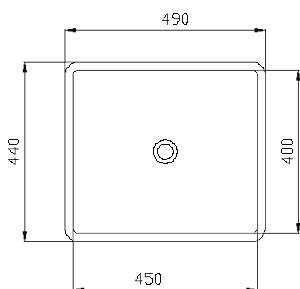
Модель ГС ОП-450
